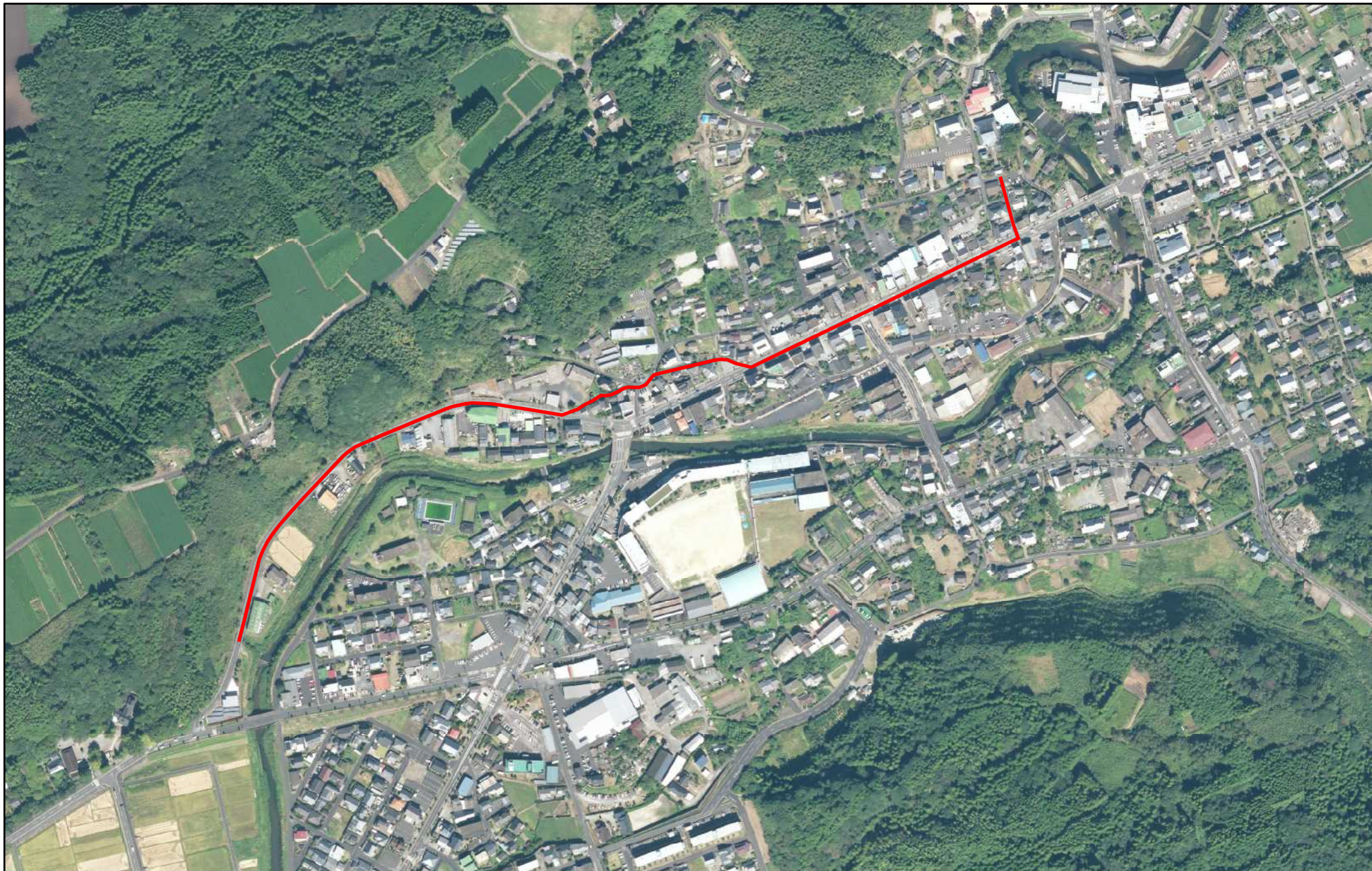
知覧都市下水路（中郡都市下水路）位置概略図 S=1:5,000
