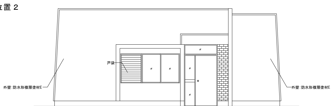
東側立面図 scale1/60
