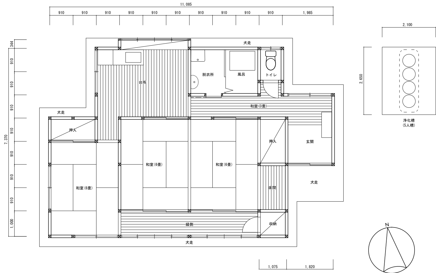
平面図 scale1/60
