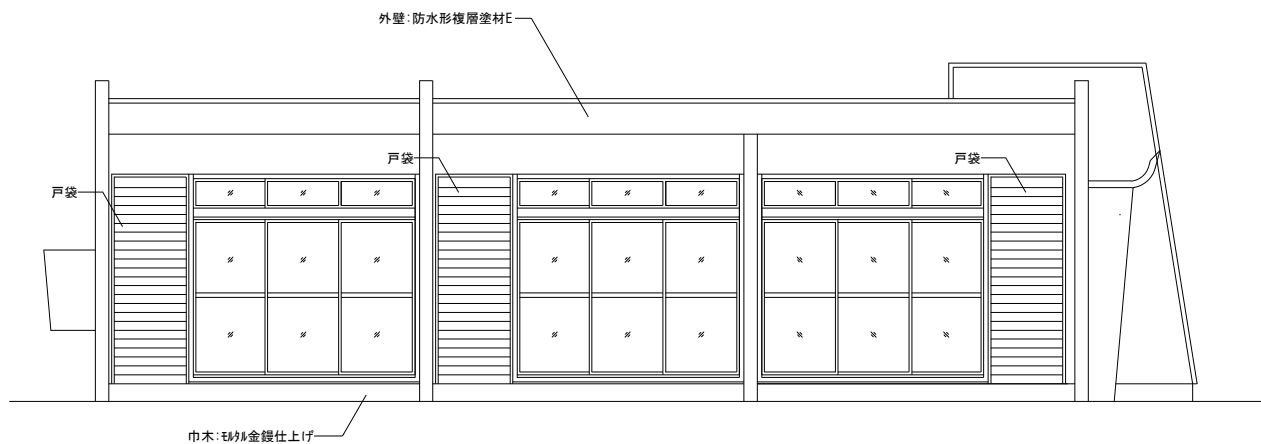
南側立面図 scale1/60
