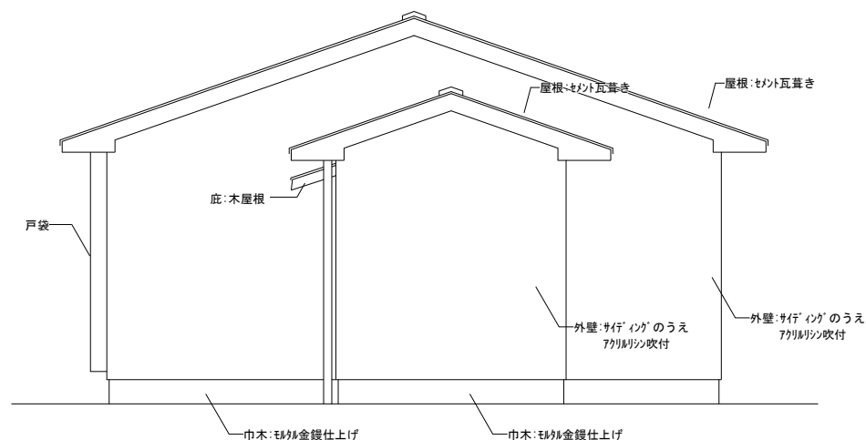
東側立面図 scale1/60
