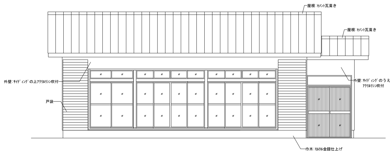
南側立面図 scale1/60
