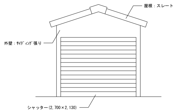
東側立面図(車庫) scale1/60
