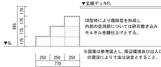
改修後階段詳細図 scale1/30
