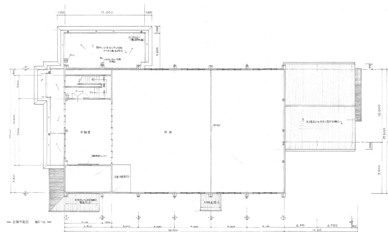
旧川辺学校給食センター 平面図（2階）
