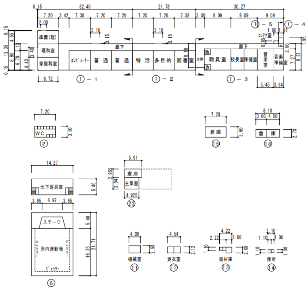
旧神殿小学校 平面図
