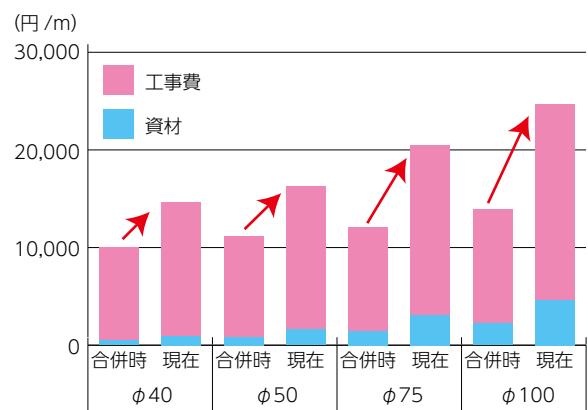
管布設m当たりの工事単価の変化
