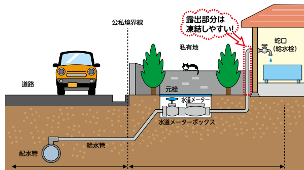
市役所水道課の維持管理範囲：お客さまの維持管理範囲（水道メーターは除く）
