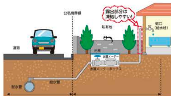
市役所水道課の維持管理範囲：皆さんの維持管理範囲（水道メーターは除く）
